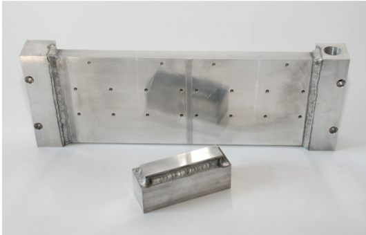
TIG/MIG robotsvejsning
